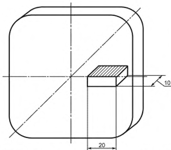
Рисунок 1 — Образец от прутка или заготовки с диаметром или длиной стороны свыше 40 \text{ мм}
